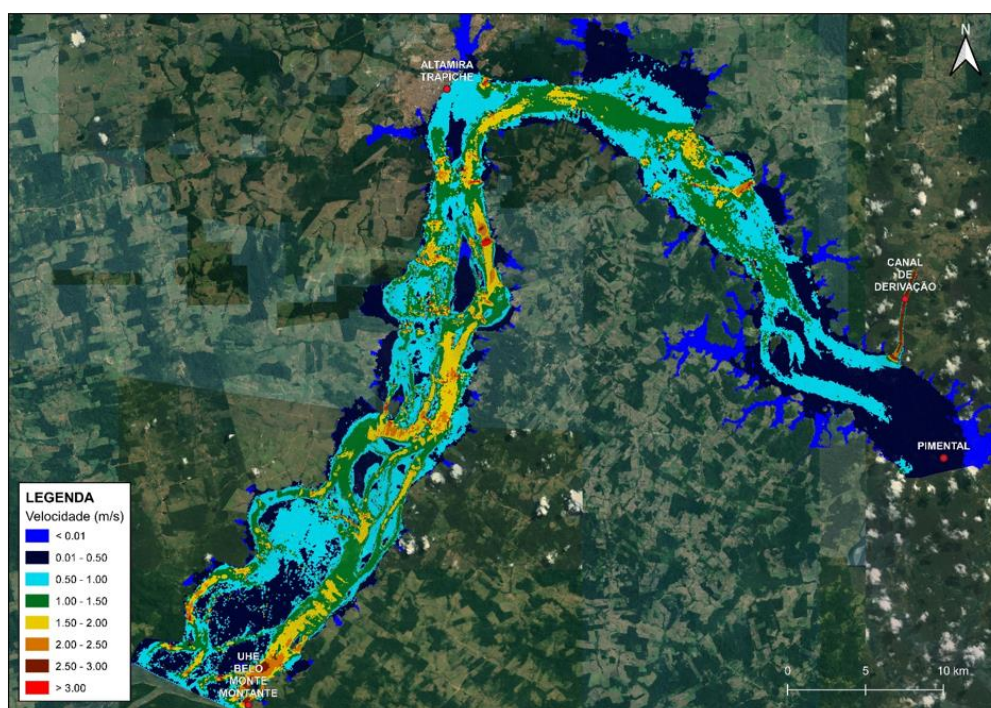
Figura 12-8 – Velocidades – 26224 m³/s
