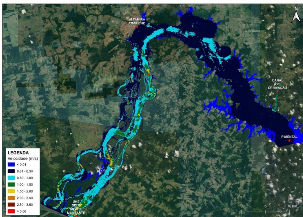
Figura 9-3 – Velocidades (8045 m³/s)
