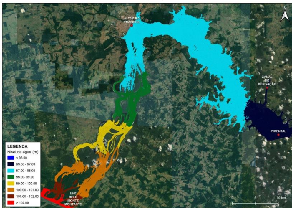
Figura 9-4 – Níveis de água (8045 m³/s)
