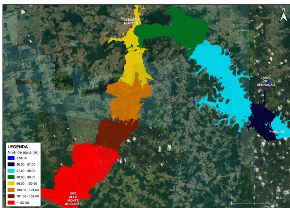
Figura 12-7 – Níveis de água – 26224 m³/s
