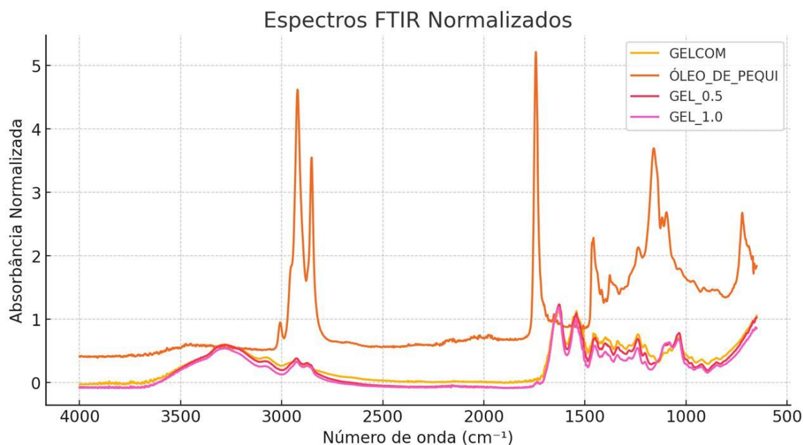
Figura S1 - Espectros normalizados dos filmes de gelatina comercial e gelatina comercial acrescidos de 0,5% e 1,0% de óleo de pequi.
